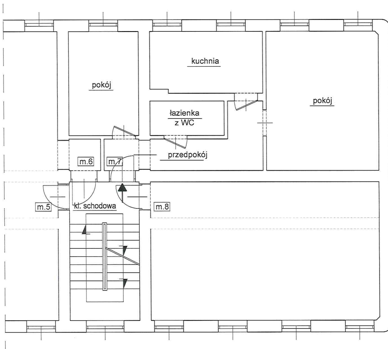
Rzut I-go piętra- fragment
